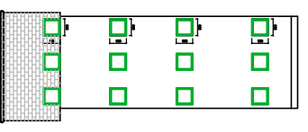
ĀTRIUM - pohľad bočný - b
